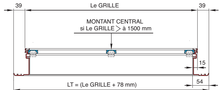
Coupe horizontale
