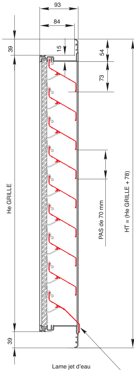
Coupe verticale
